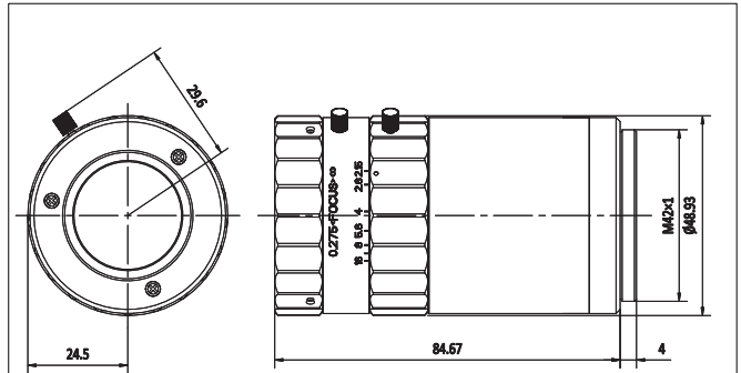
大靶面高分辨率短波近红外镜头 高分辨率 大光圈设计 紧凑型设计 800-1800nm
